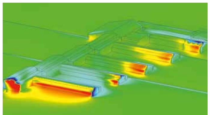
CFD-Analyse, Windrichtung: S
